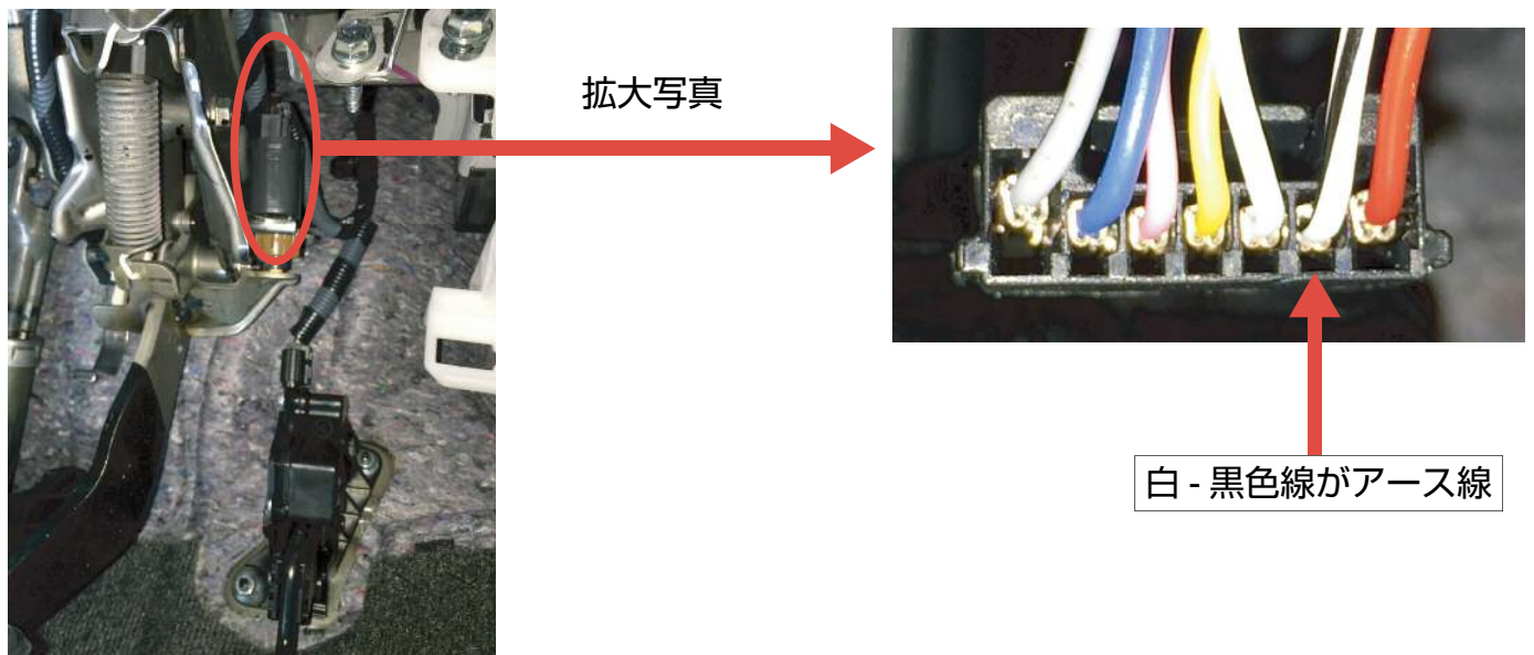
配線側から見たコネクタ配線位置
