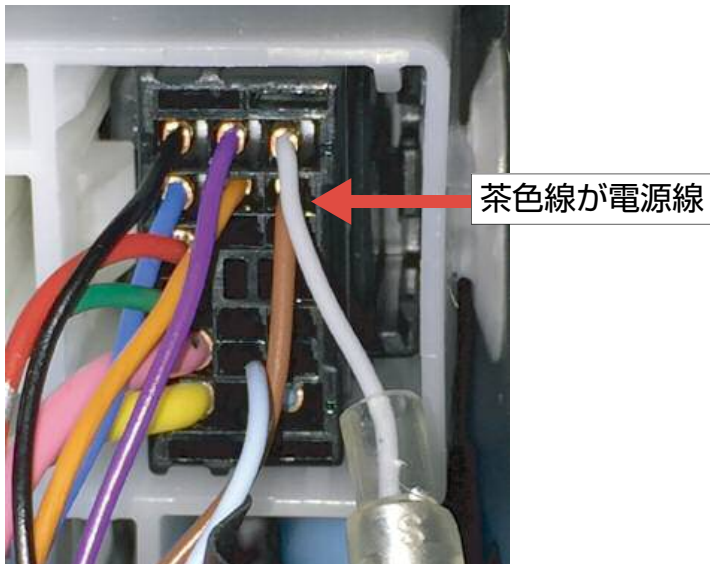
配線側から見たコネクタ配線位置
