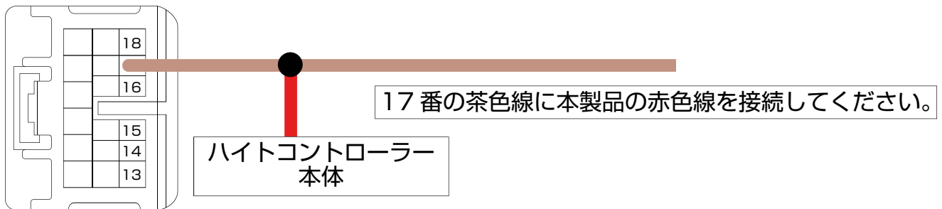
配線側から見たコネクタ配線位置
