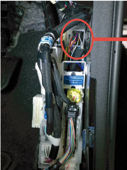
配線側から見たコネクタ配線位置
