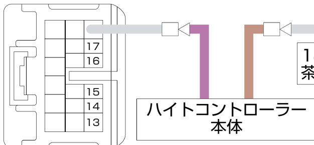
配線側から見たコネクタ配線位置
