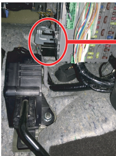
配線側から見たコネクタ配線位置
